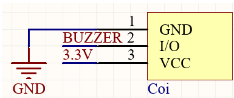
Hình 3.10 Sơ đồ nguyên lý khối cảnh báo
