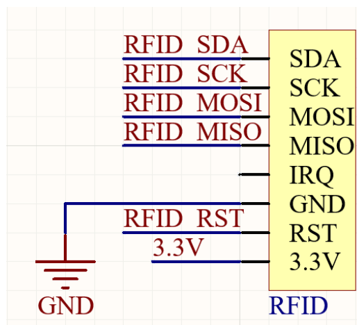
Hình 3.6 Sơ đồ nguyên lý khối RFID RC522
