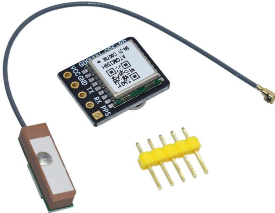
Hình 3.3 Module GPS ATGM336H
