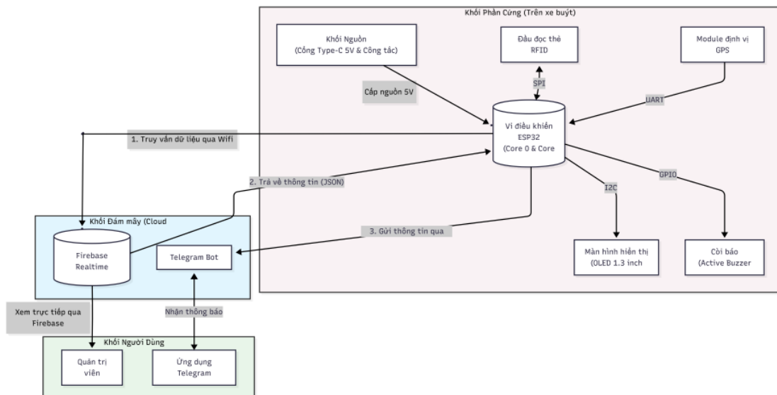
Hình 2.1 Sơ đồ khối kiến trúc hệ thống
